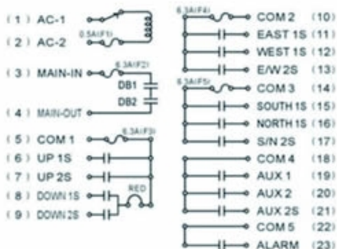
SAGA1-K2接线图
