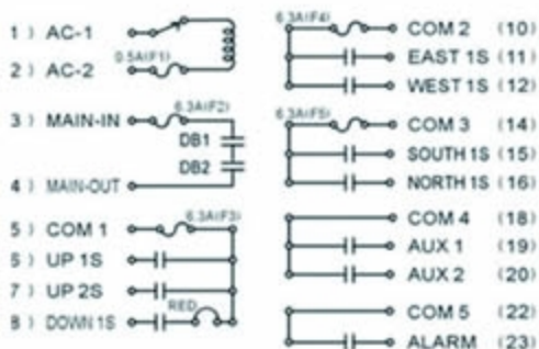
SAGA1-K1接线图
