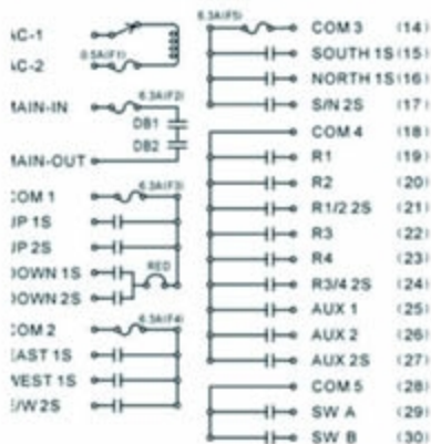
SAGA1-K4接线图
