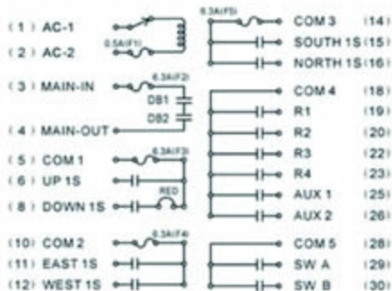
SAGA1-K3接线图
